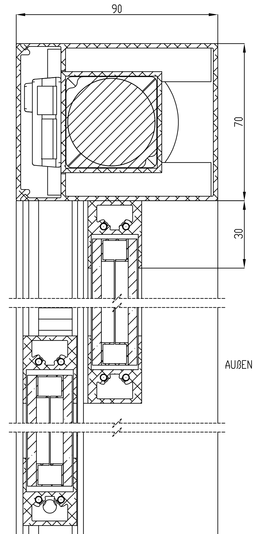
B-B 1 : 1
