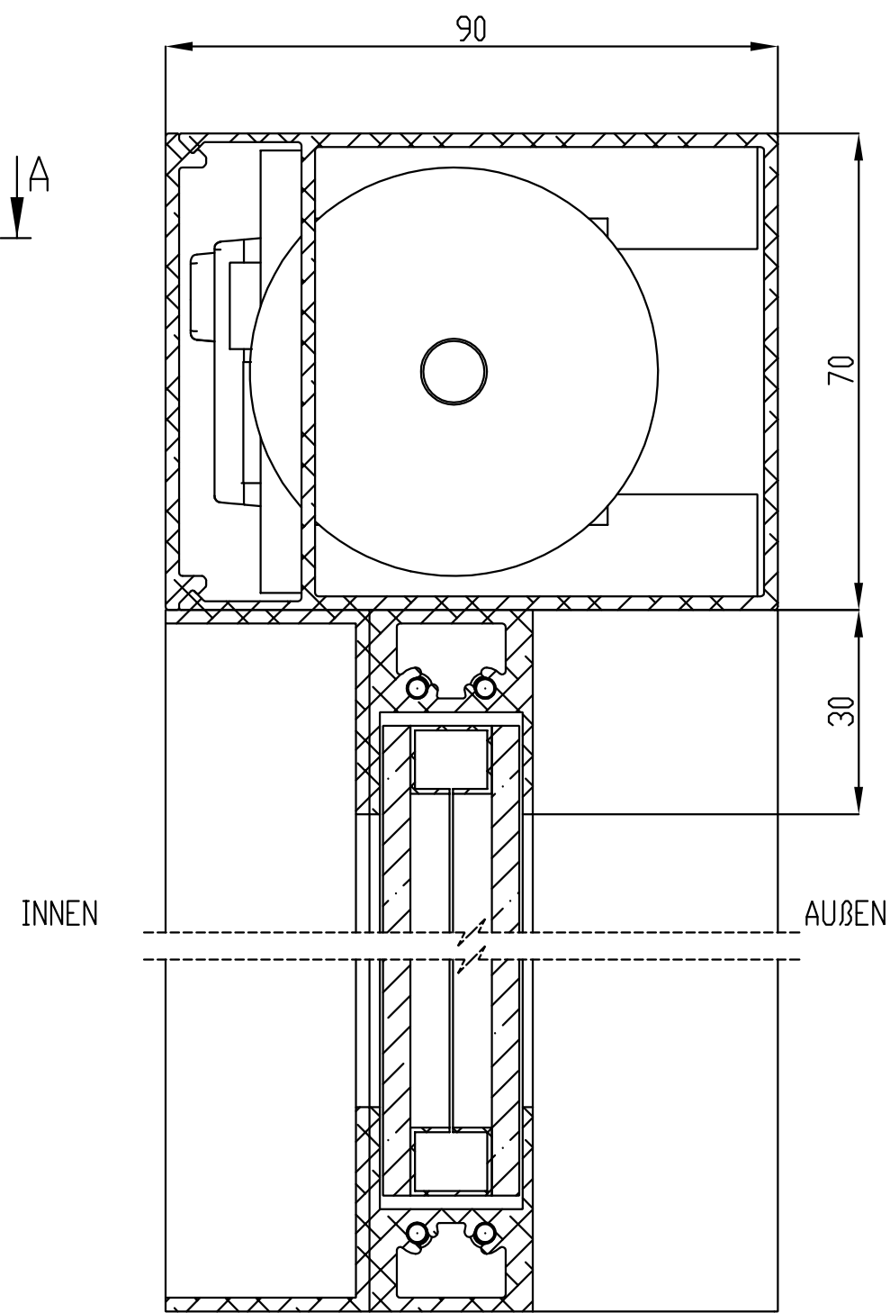
C-C 1 : 1
