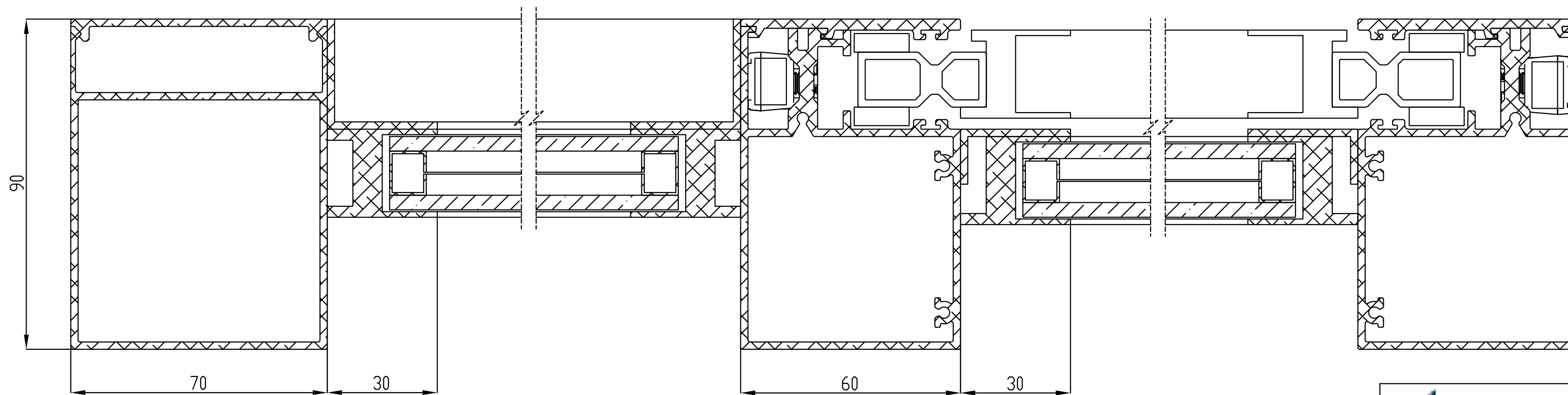
A-A 1 : 1
