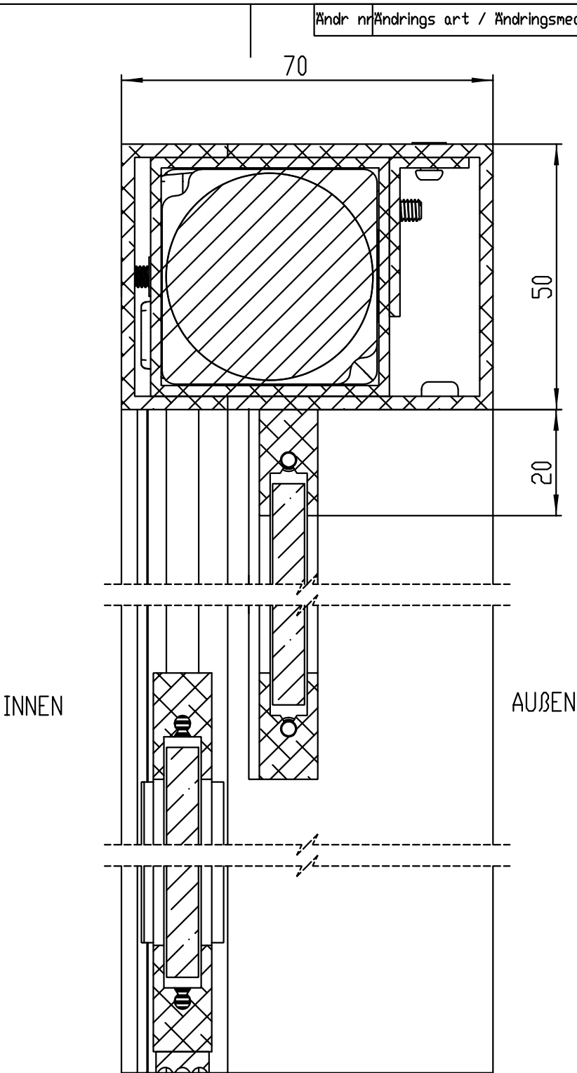
B-B 1 : 1
